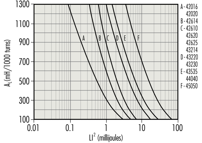
E CORES
